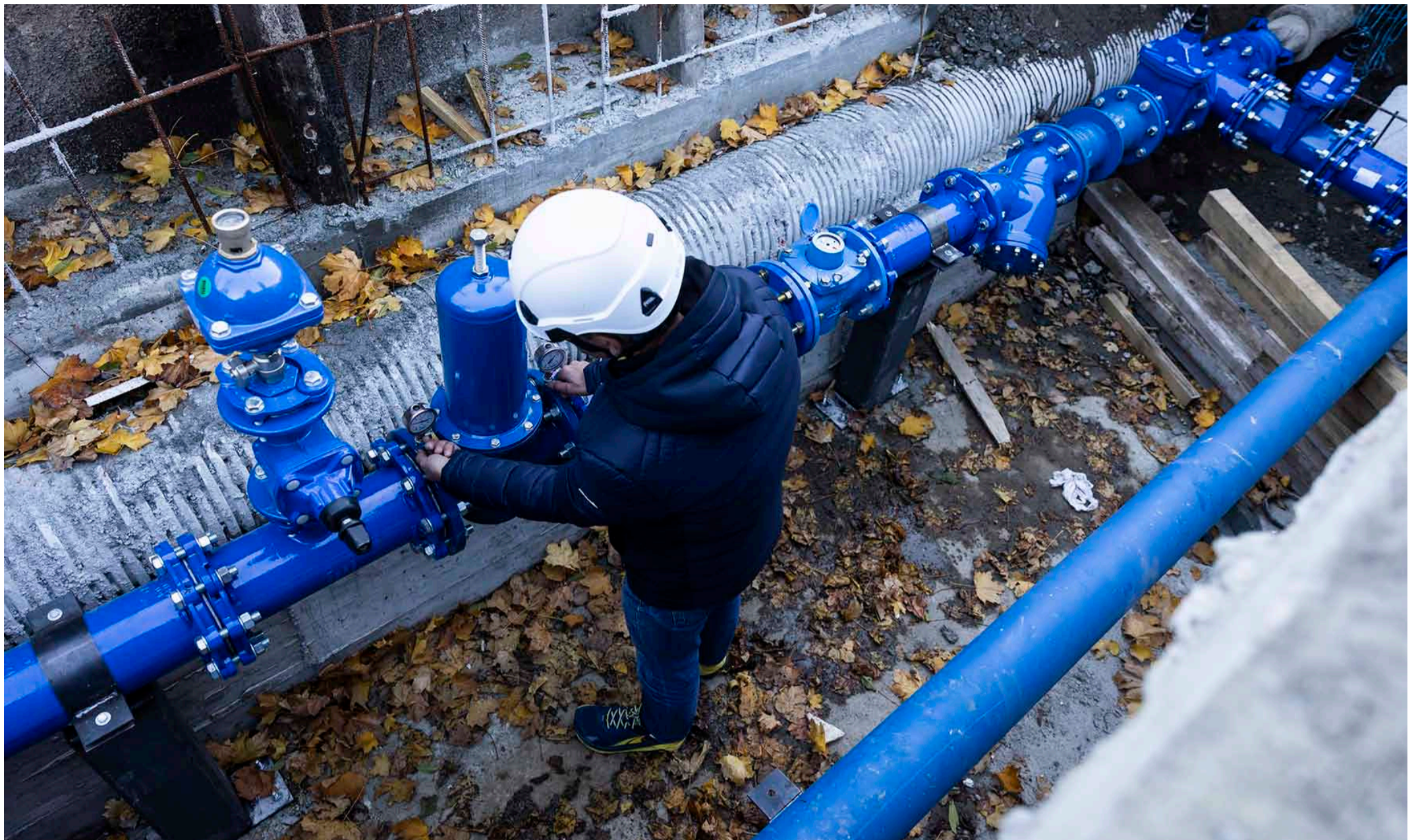
Els treballs de sectorització i digitalització de la xarxa d'aigua potable a Andorra la Vella.
